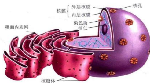
图 8-3 核被膜基本结构示意图
