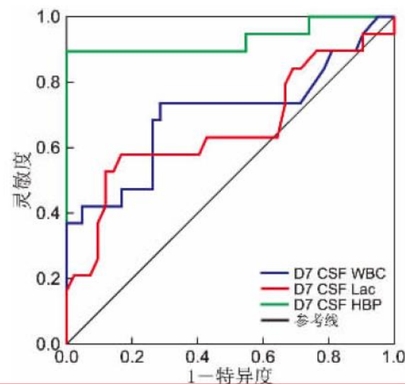
图 3 脑脊液白细胞、乳酸、HBP 预测预后的 ROC 曲线
